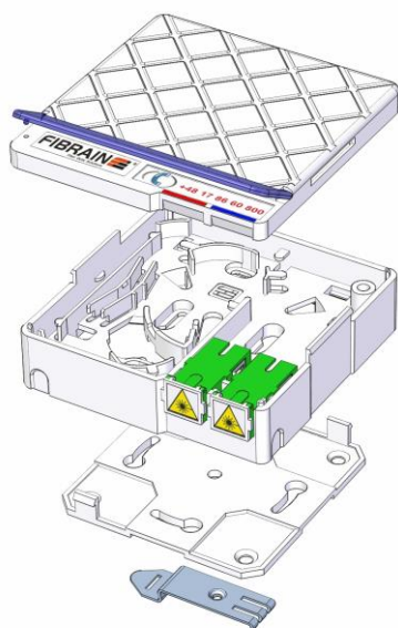
Budowa puszki
